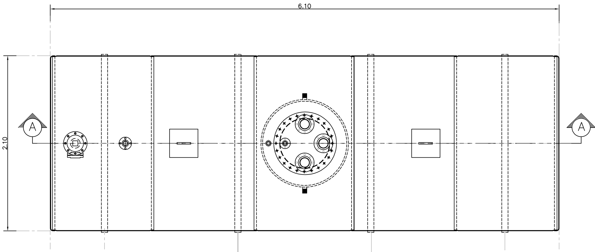
แปลนการสร้างถังใต้ดินผนังสองชั้น ขนาด 20,000 ลิตร (SUBMERSIBLE)
